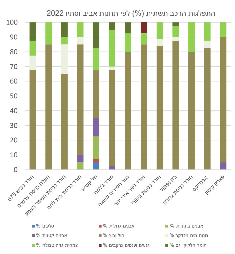
איור 2. התפלגות הרכב תשתית לפי אחוז כיסוי בנחל קישון. הערכים בטבלה הינם ממוצעים שחושבו עבור ניטור אביב-סתיו 2022.
