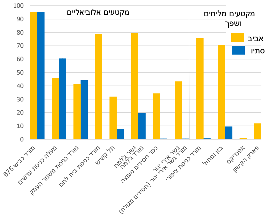
איור 6. התפלגות האחוז היחסי של ימוששים בין מקטעי הדיגום האלוביאליים, המליחים והשפך בנחל הקישון באביב וסתיו 2022.
